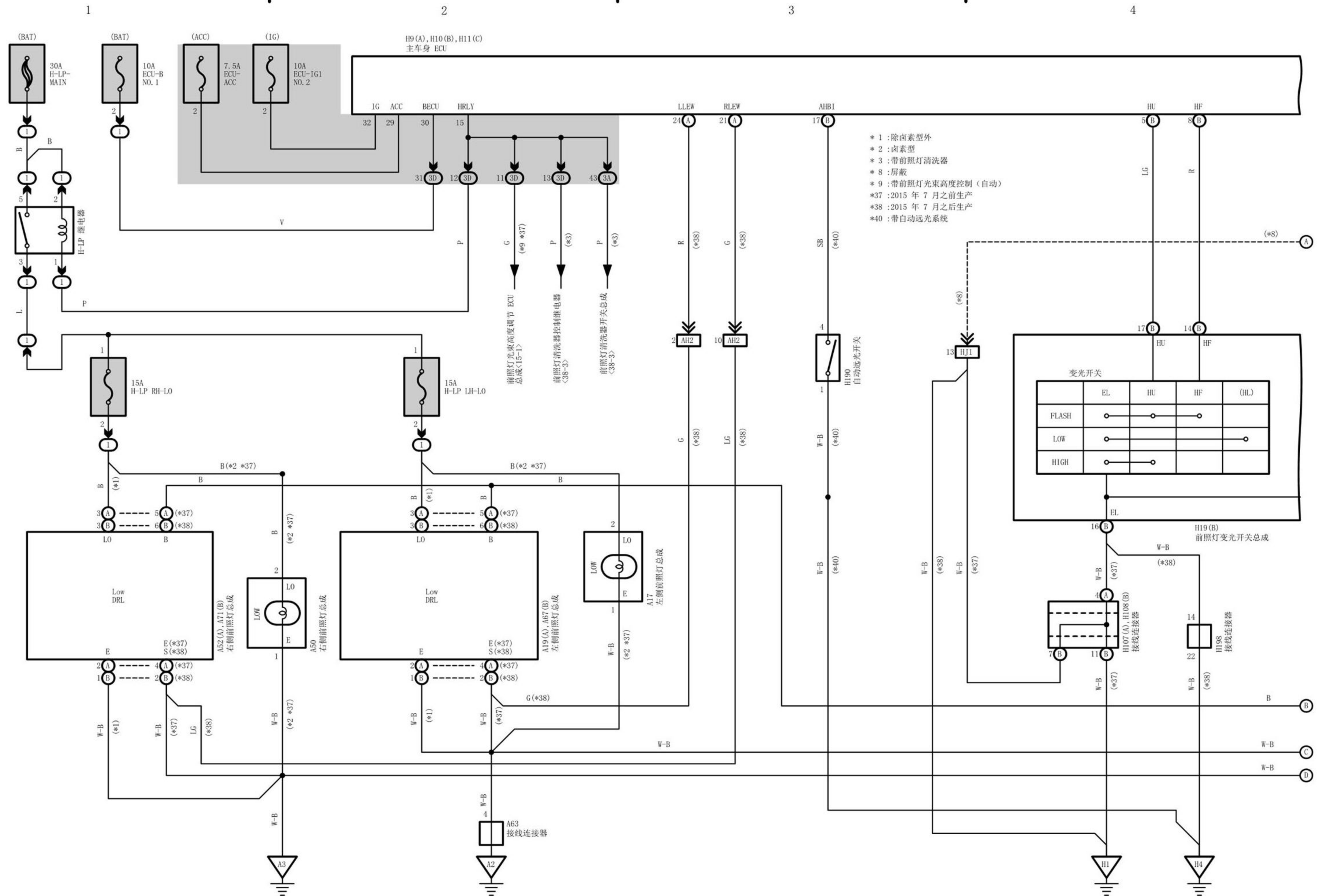
前照灯（右驾驶车型）
